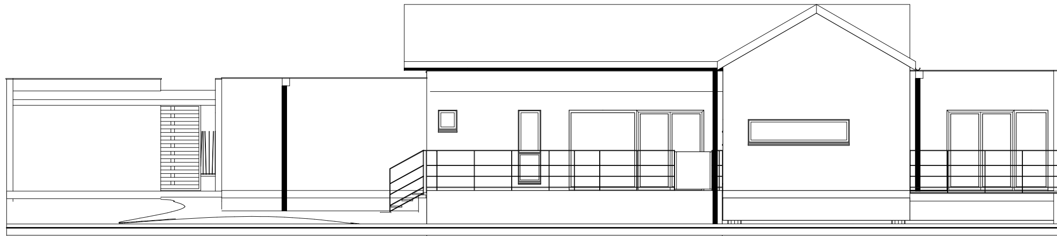
ELEVATION SUD
