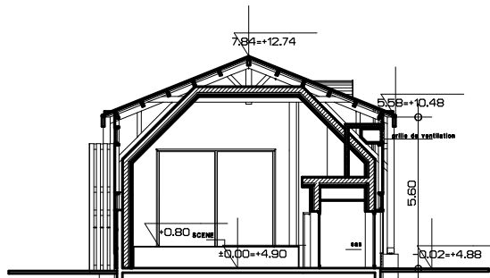
COUPE/ESPACE SCENIQUE
